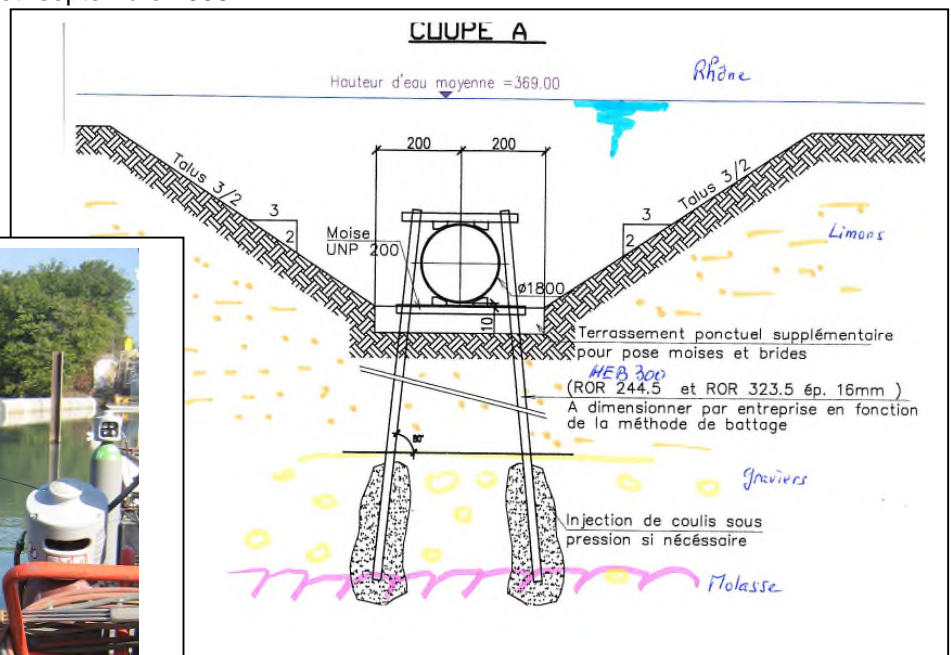
Coupe type – Zone draguée
