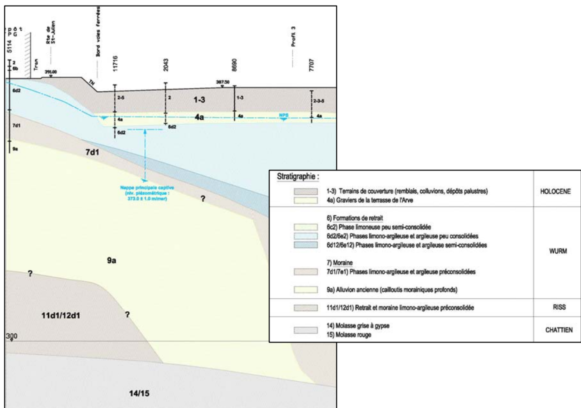
Extrait du profil géotechnique interprétatif n°4 Bande verte
