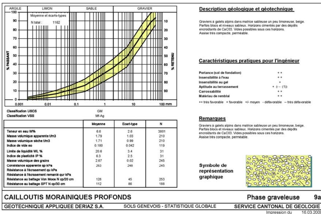
Exemple d'une fiche signalétique : Alluvion ancienne phase graveleuse 9a
